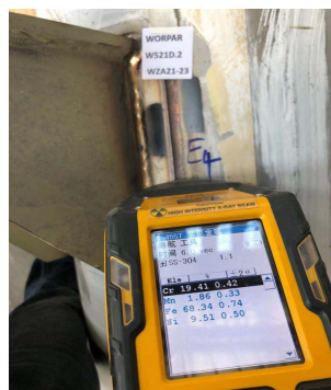
WELD E4
