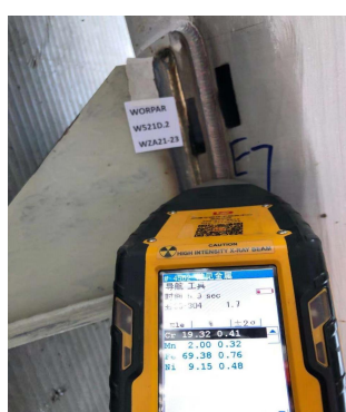
WELD E7
