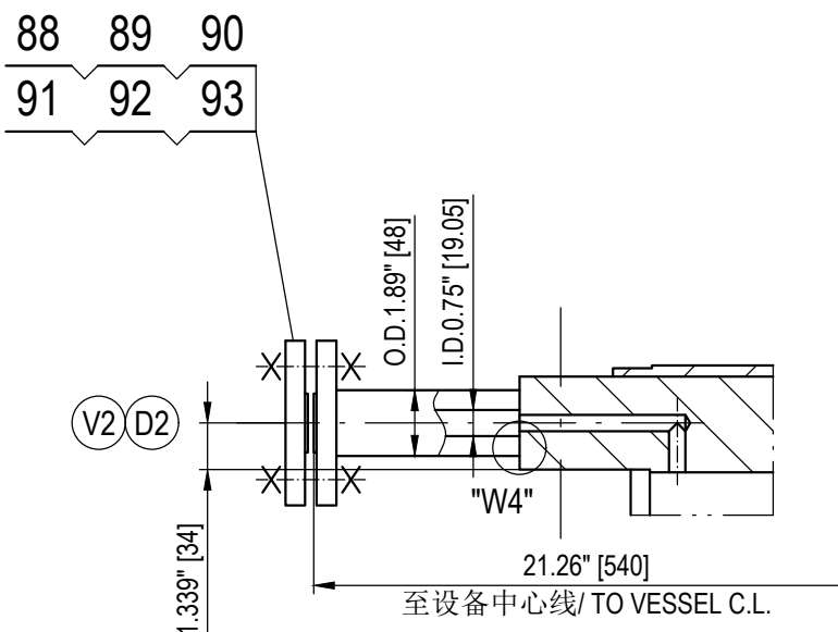
接管V2,D2详图 DETAIL OF NOZZLE V2,D2
