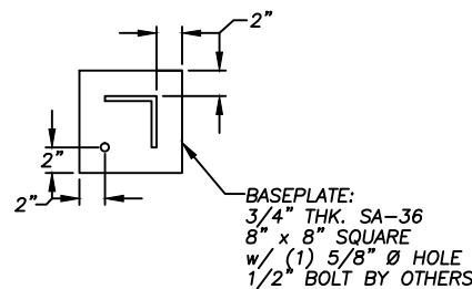
LEG DETAIL SCALE: N.T.S. (3) REQ'D
