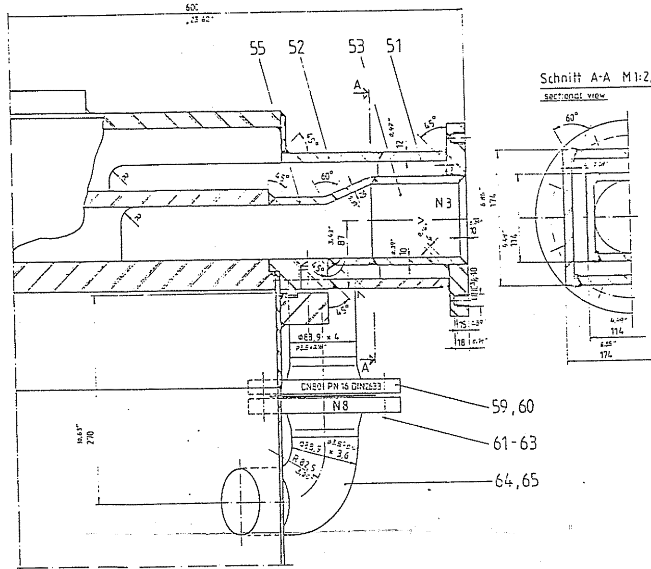
Tangentialstützen oben N3 M. 1:2,5 top tangential flange N3 scale 1:2.5
