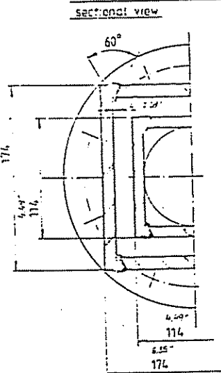
Schnitt A-A M.1:2,5 SECTIONAL VIEW
