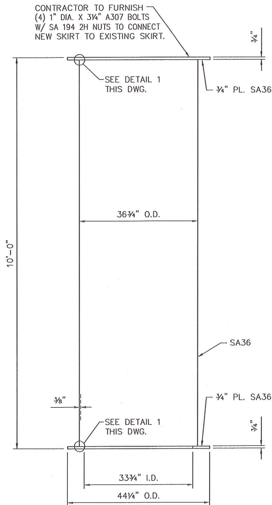
ELEVATION SCALE: 3/4" = 1'-0"
