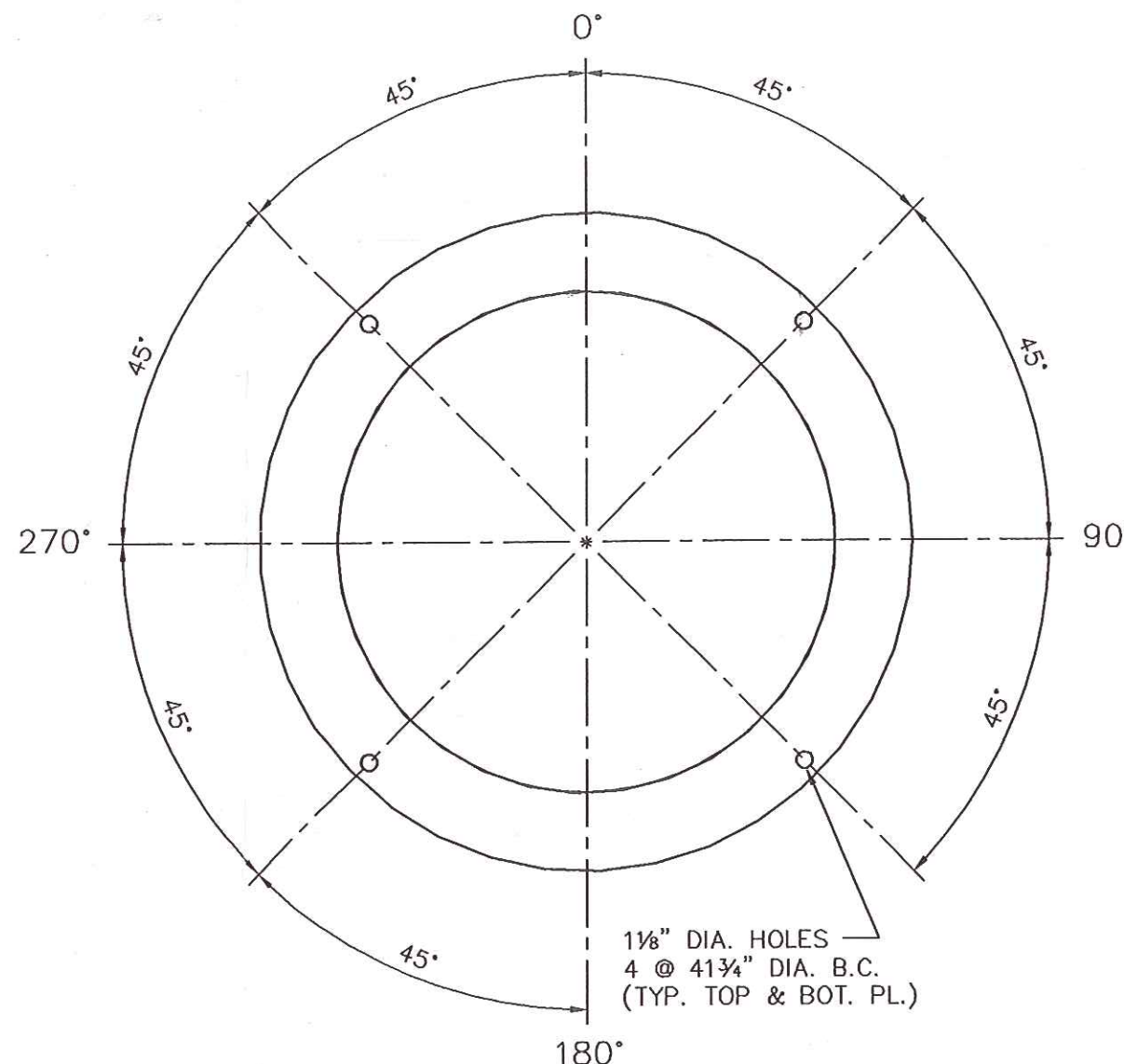
PLAN SCALE: 1" = 1'-0"
