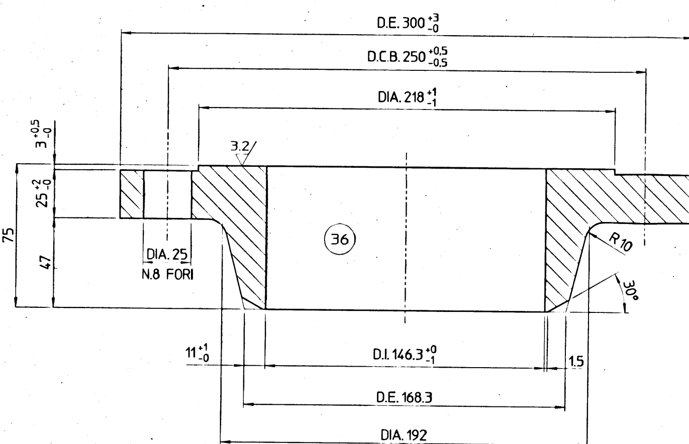
FLANGIA DN 150 PN 25 UNI 2283-67 BOCCELLO MARCA 'E'
