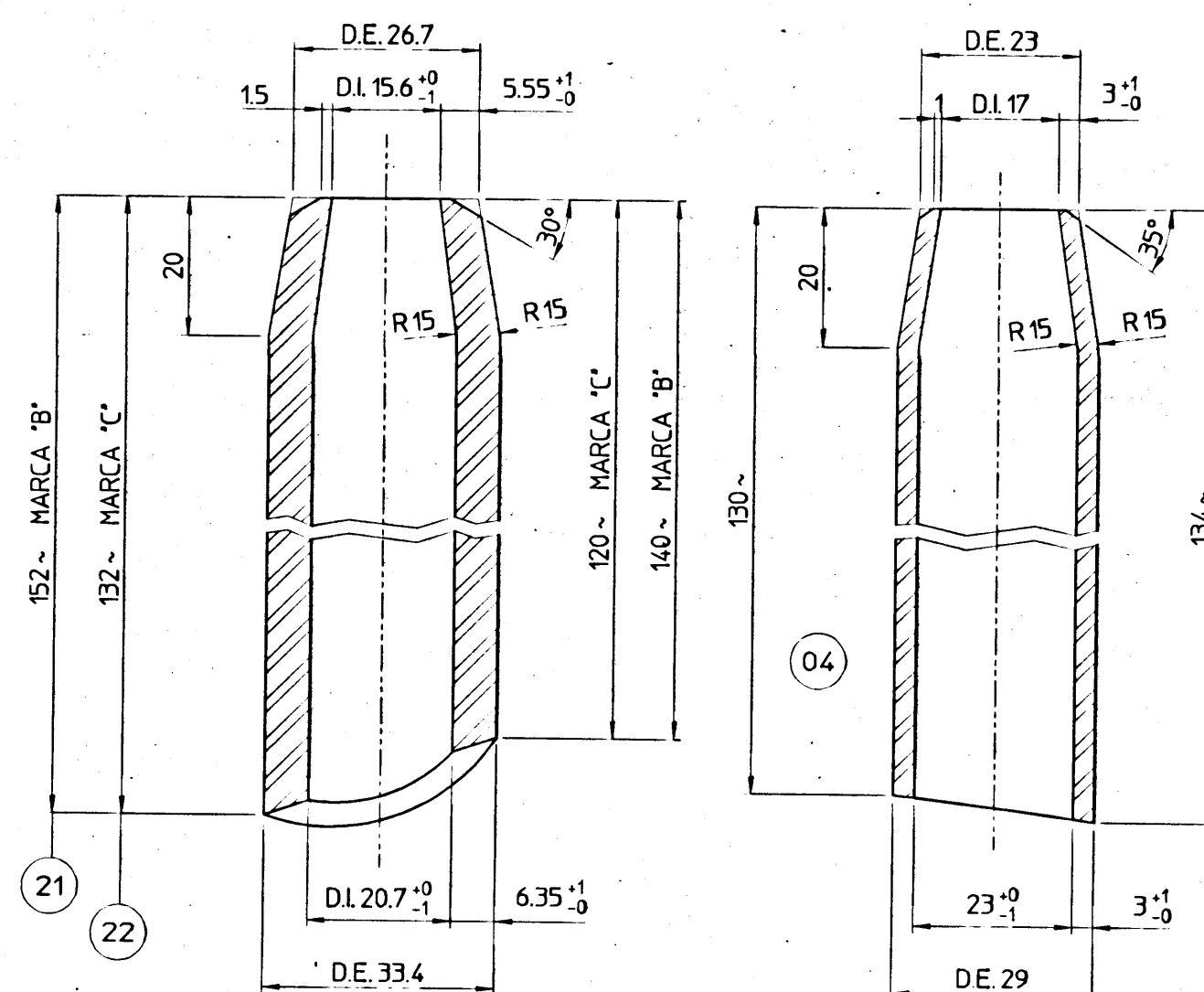
N.2 TRONCHETTI RICAVATI DA TONDO BOCCELLI MARCA 'B-C'
