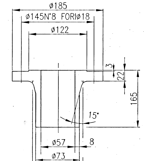
△ PART.FLANGIA LWN "D" (108)
