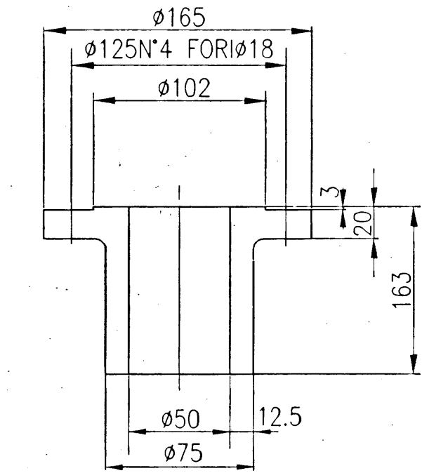
PART.FLANGIA LWN "G" (112)
