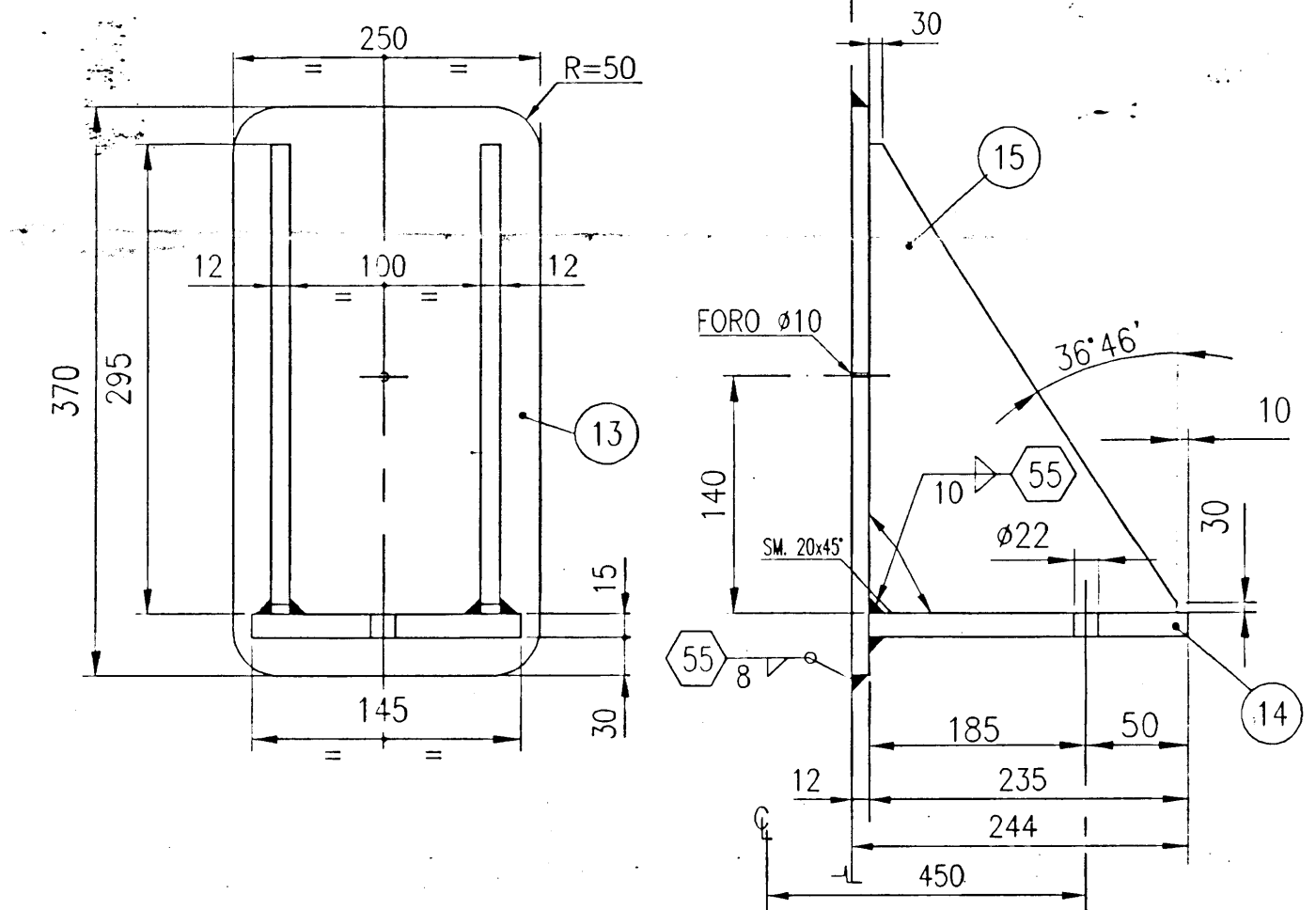
PART. ORECCHIA DI SOLLEVAMENTO (N°1PEZZO)
