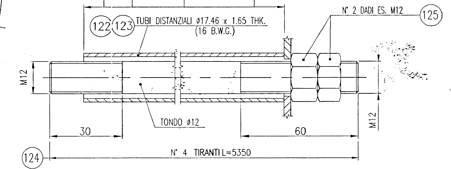
PART. SELLE DI SOSTEGNO (N°2 PEZZI)
