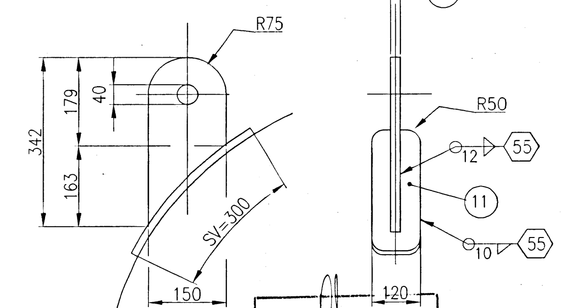
PART. ORECCHIA DI SOLLEVAMENTO (N°1PEZZO)
