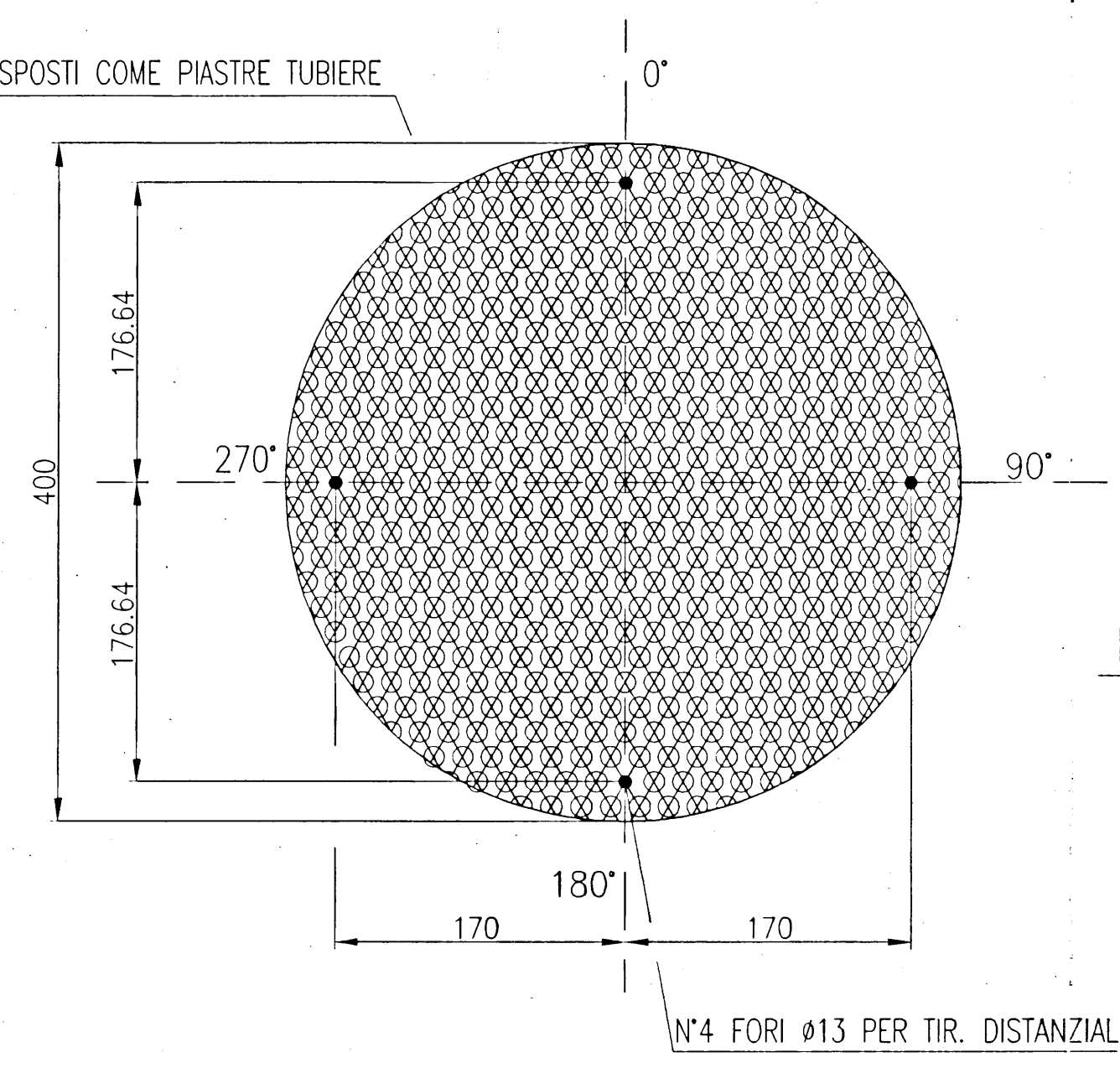
△ PART.FLANGIA LWN "D" (108)
