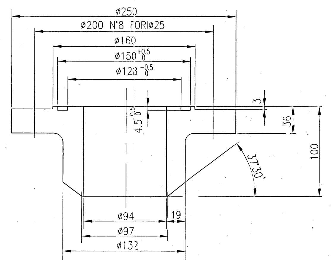
PART.FLANGIA LWN "A" (106)
