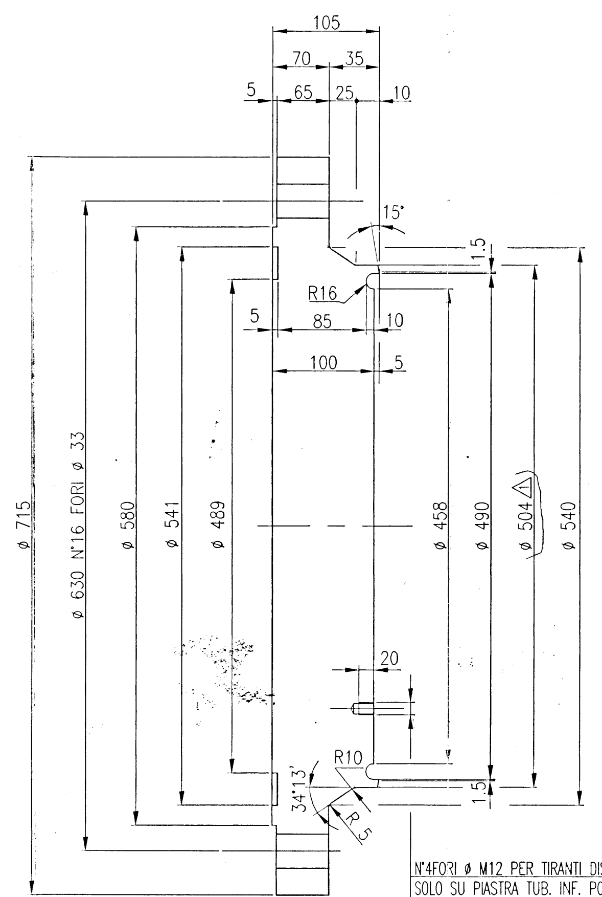
(17) DIAFRAMMA TIPO "B" (N°5 PEZZI SP.6)
